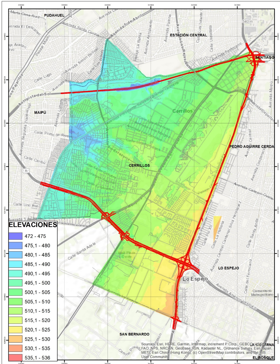
Figura 4 Plano de elevaciones comuna de Cerrillos
